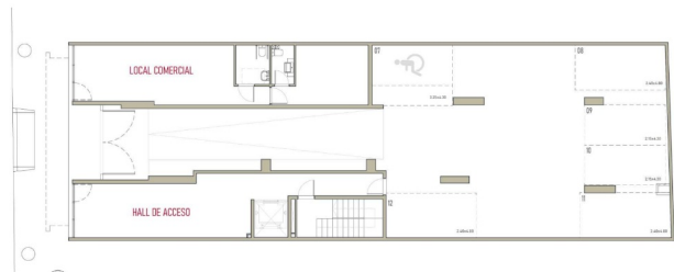
PLANTA BAJA Hall de acceso, Local comercial, Garajes.
