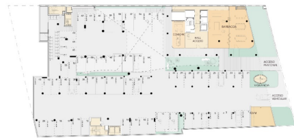
> Planta Acceso por Sanguinetti, Garajes, Barbacoa, Cowork y Gym
